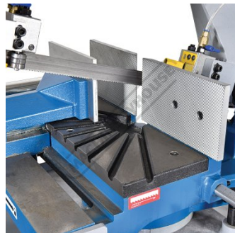
Dual Mitre Slots
